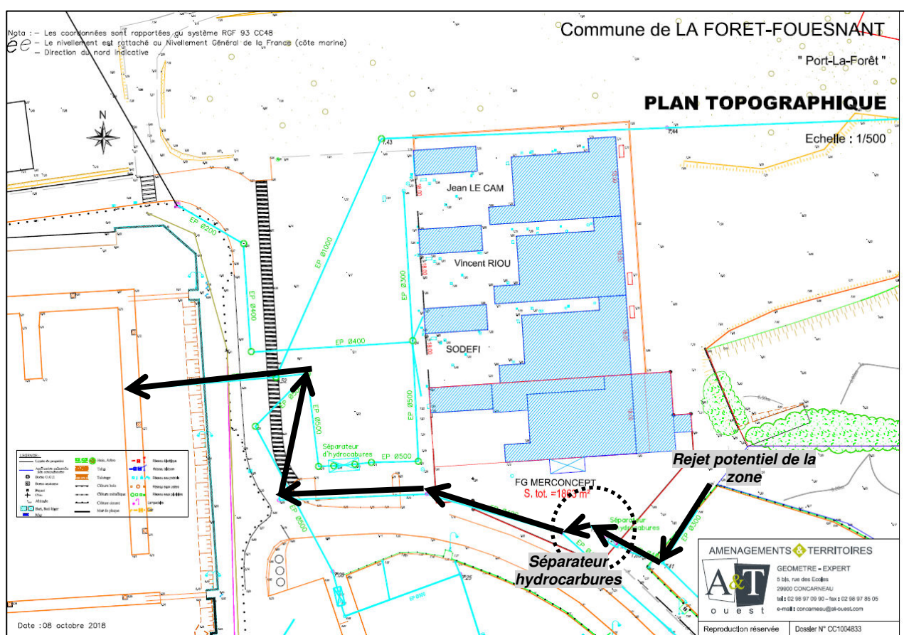
Figure 10 : Réseau en aval de la zone urbanisable n°9
