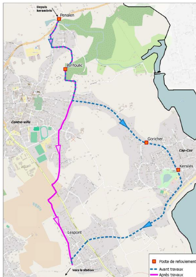
Figure 6 : Synoptique de la modification sur le transfert des eaux usées au niveau des postes de Kervransel, Pen Al Lenn et Penfoullic
