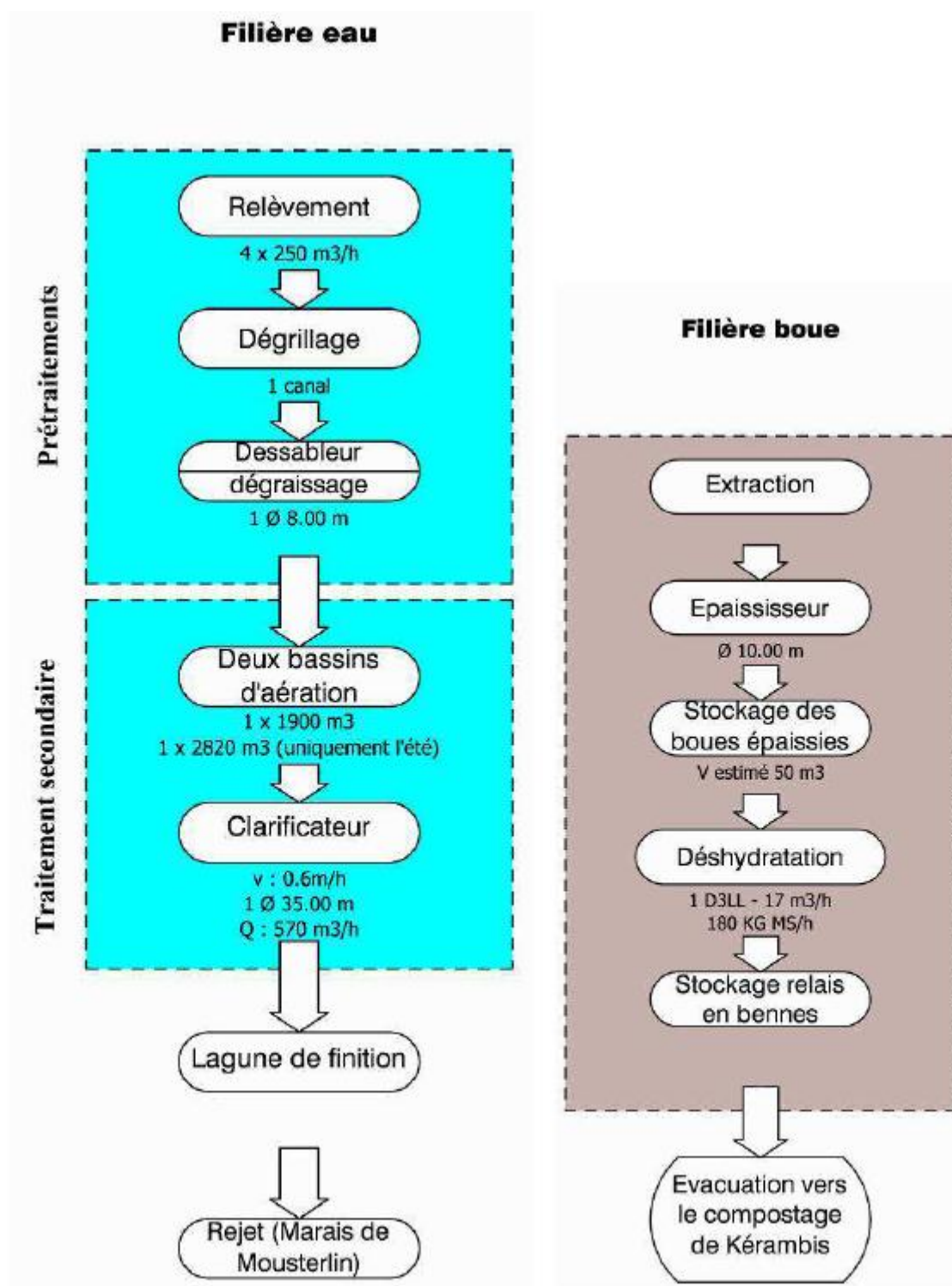
Figure 7 : Synoptique des filières « eau » et « boues »
